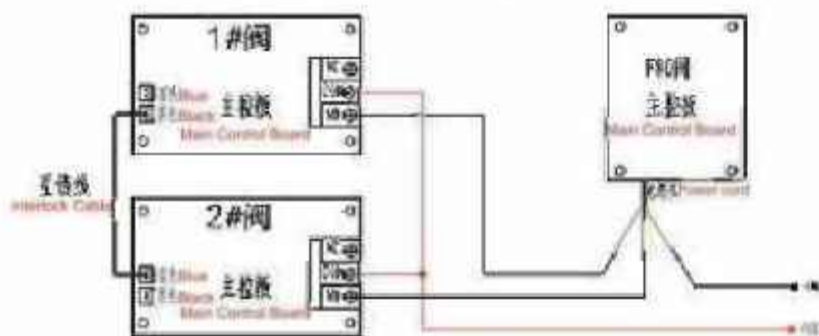
一用一备系统接线图
